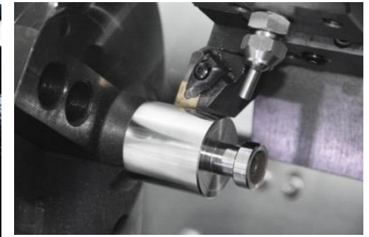
CNC strugovi
