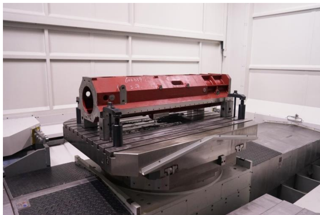
Ram portalnog obradnog centra
